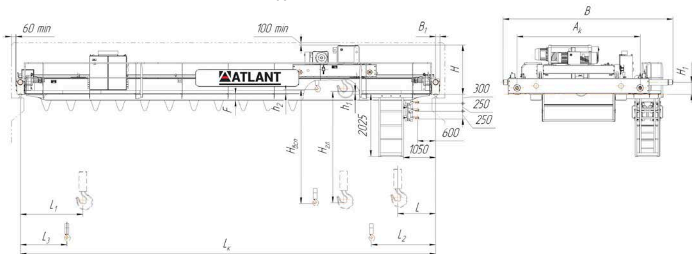
Кран мостовой опорный электрический двухбалочный г/п 20т и 5т
