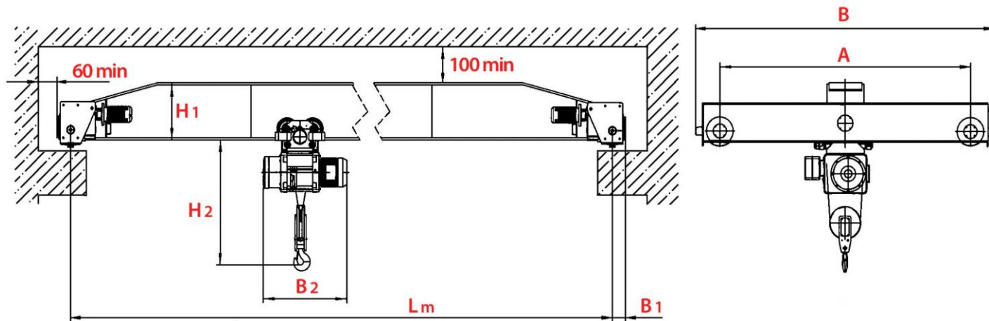
Кран мостовой опорный электрический КМОЭ-5
